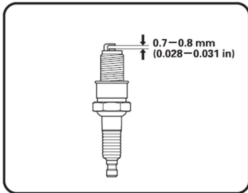
Abb. 8-6 Zündkerze prüfen
