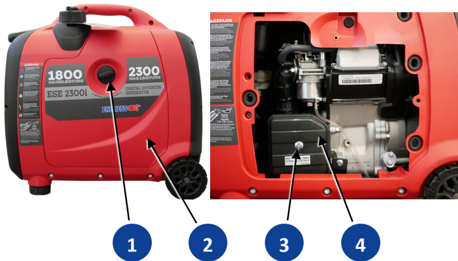
Abb. 8-4 Luftfilter hinter Wartungsklappe (entfernt)
