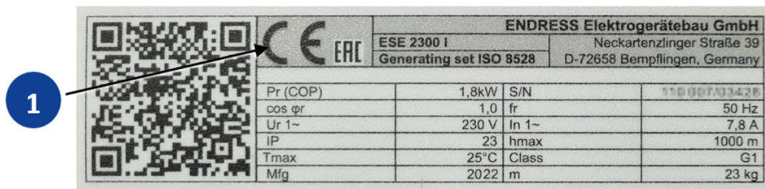
Abb. 3-1 Beispiel Typenschild
